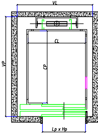
DIMENSIONI DI INGOMBRO IN MM VANO MURATURA
